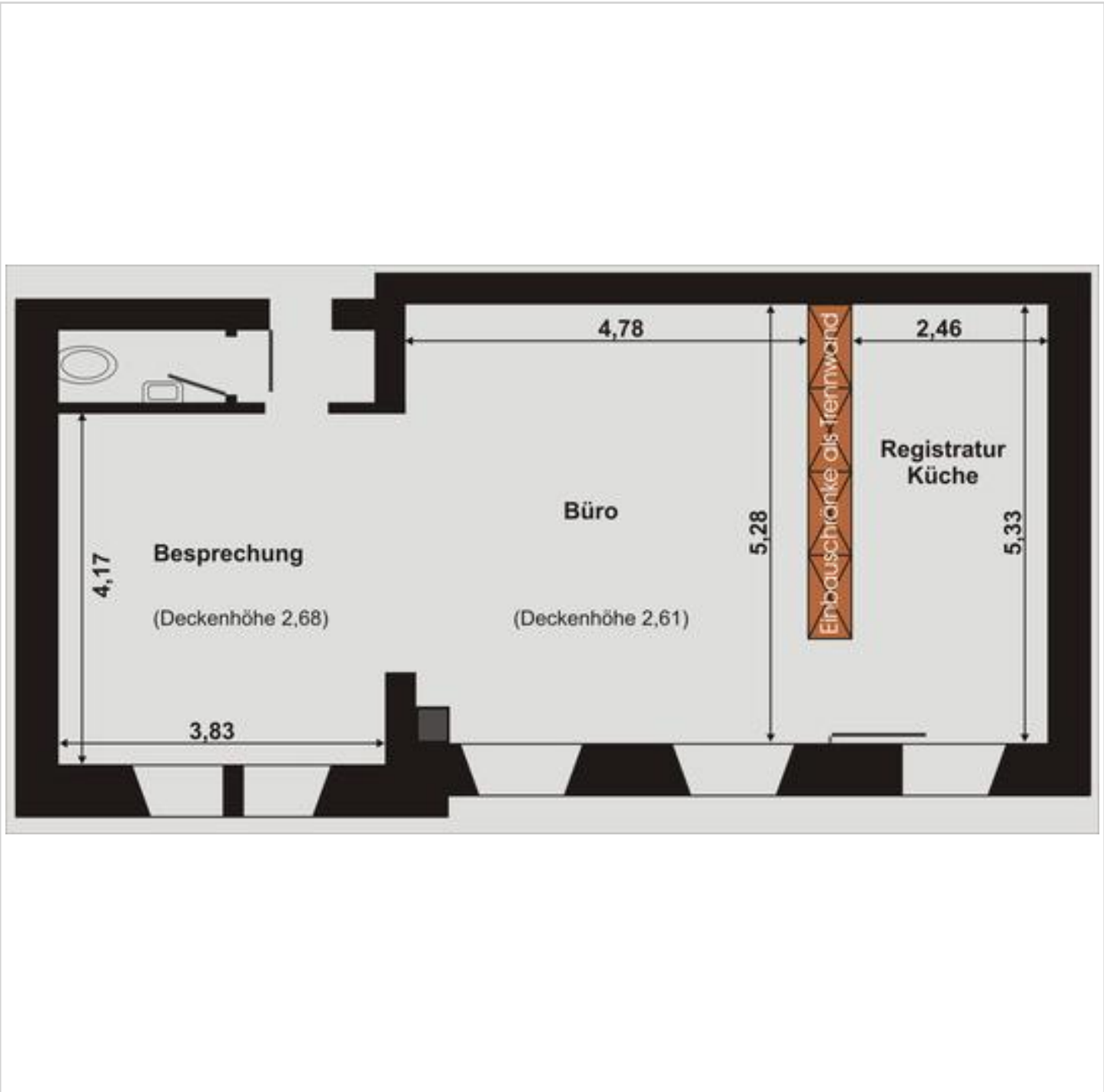
Büro Grundriss vermasst
